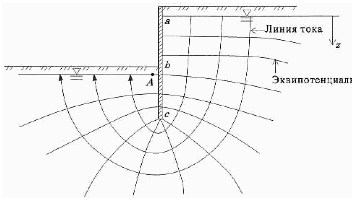
Рисунок 9.3 - Фильтрация в котлован при несовершенной ПФЗ
