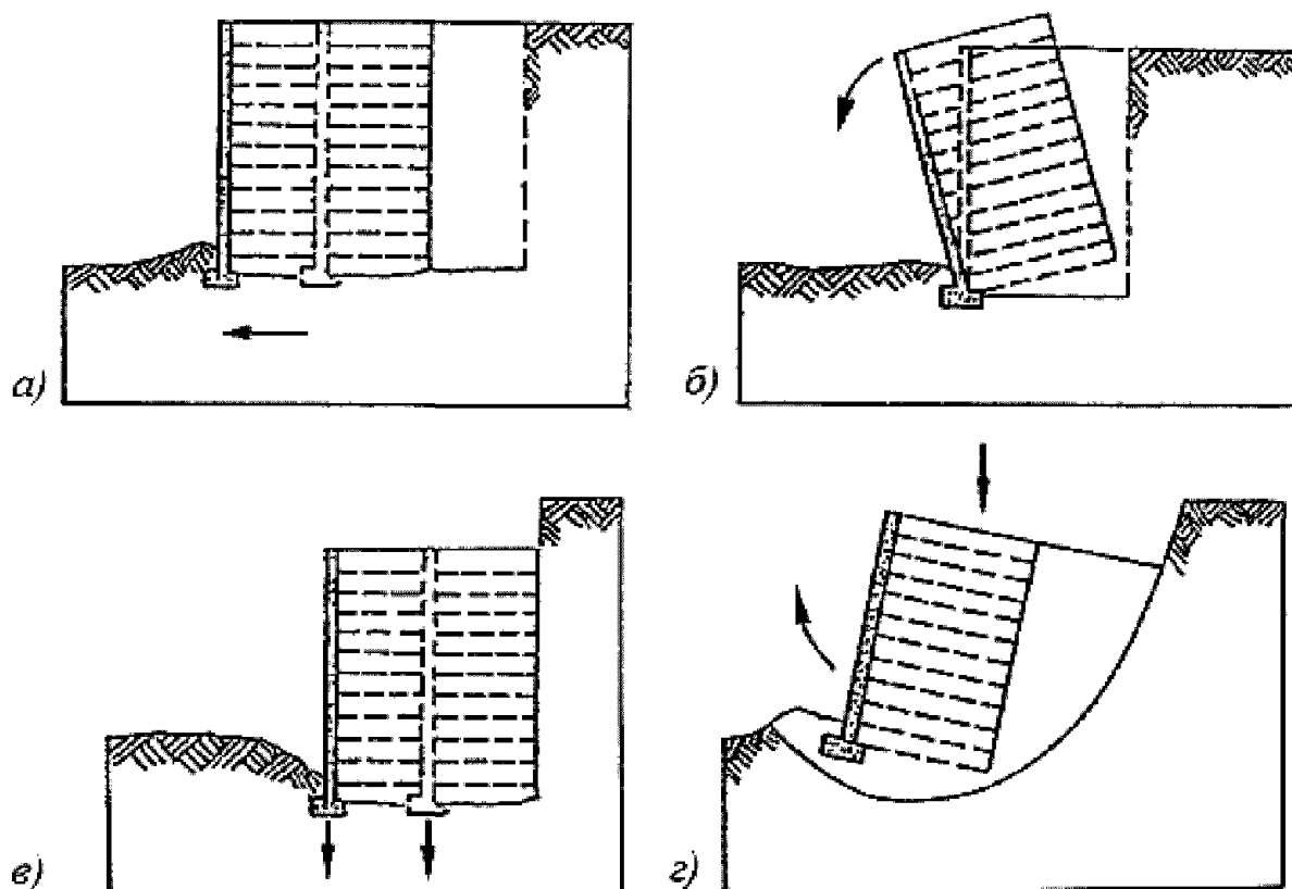
а - сдвиг по подошве; б - опрокидывание; в - потеря несущей способности подстилающего массива грунта; з - глубинный сдвиг
