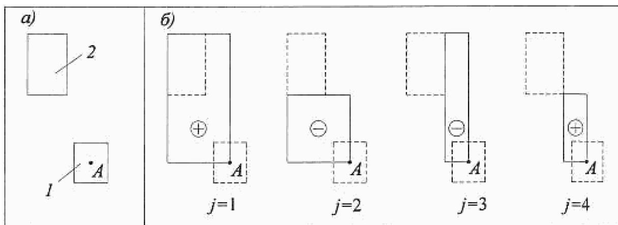
a - схема расположения рассчитываемого 1 и влияющего фундамента 2; b - схема расположения фиктивных фундаментов с указанием знака напряжений \sigma_{zp,cj} в формуле (5.21) под углом j -го фундамента
