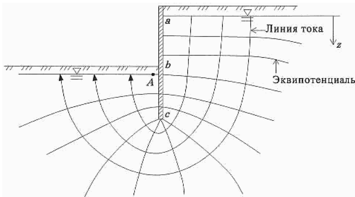
Рисунок 9.3 - Фильтрация в котлован при несовершенной ПФЗ
