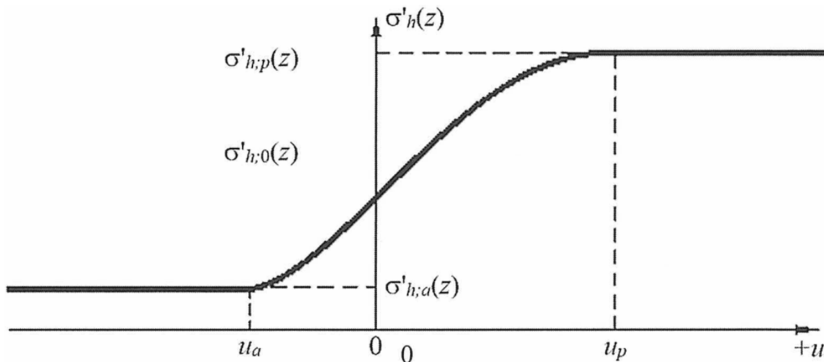
Рисунок 9.1 - Зависимость величин бокового давления грунта
